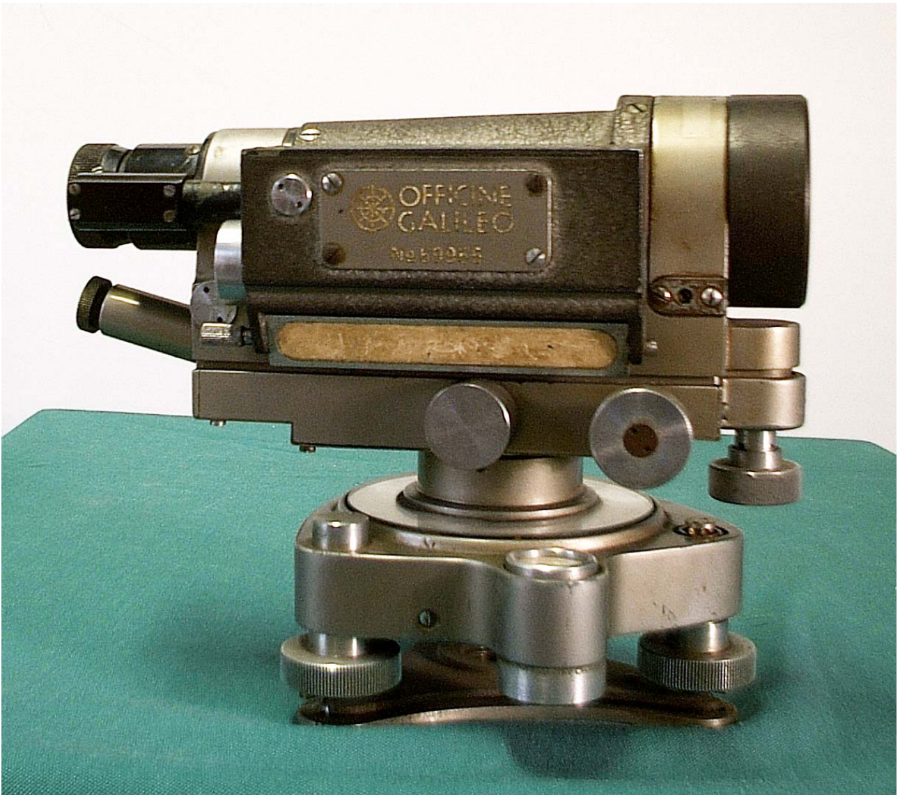
N° inventario 149 – Livello Galileo M6 con cerchio Hz sessagesimale matr. 69955 (1941)
