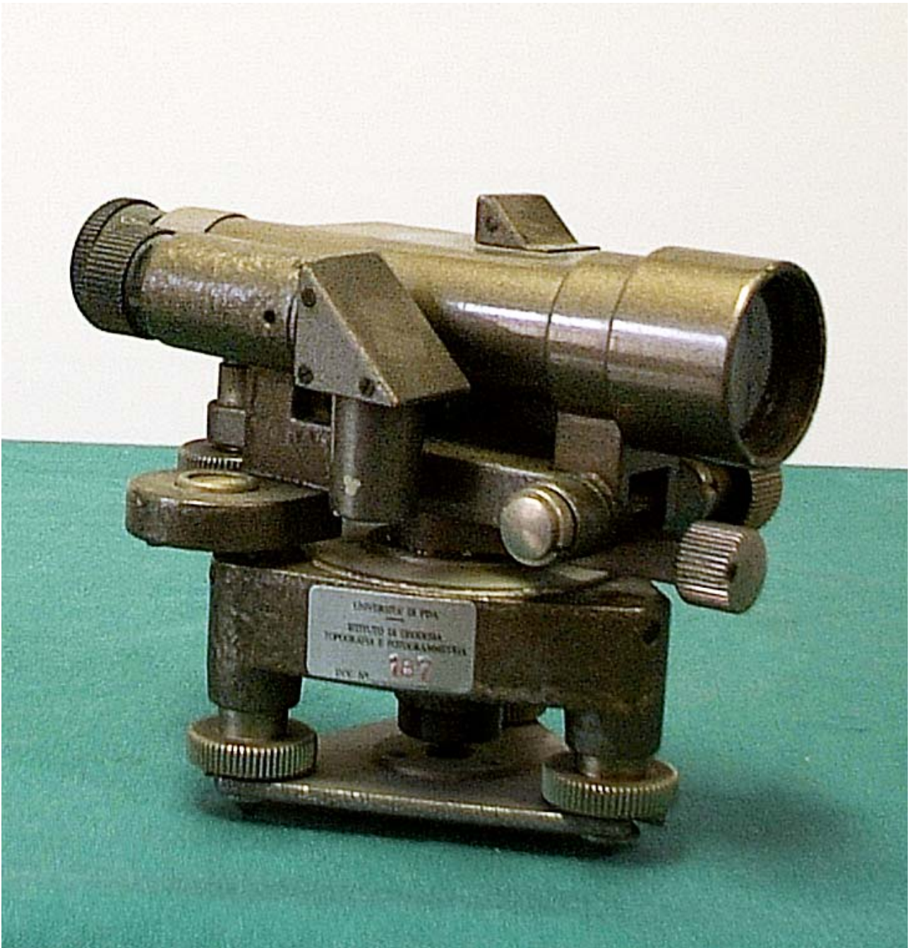
N° inventario 187 – Livello O.M.I. da cantiere matr. 77a-1605 (1948)
