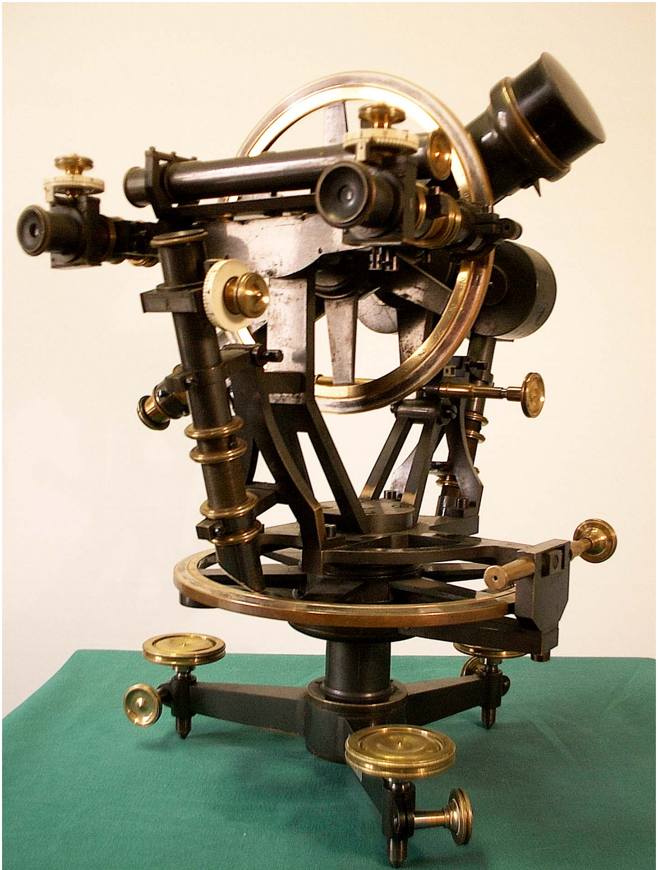
N° inventario 252 – Teodolite Salmoiraghi tipo Stark (1956)
