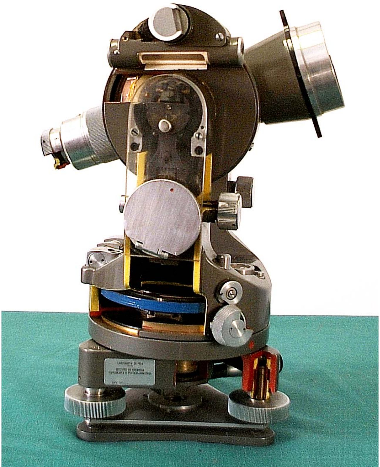
N° inventario 280 – Tacheometro sezionato Salmoiraghi mod. 4150 (1957)
