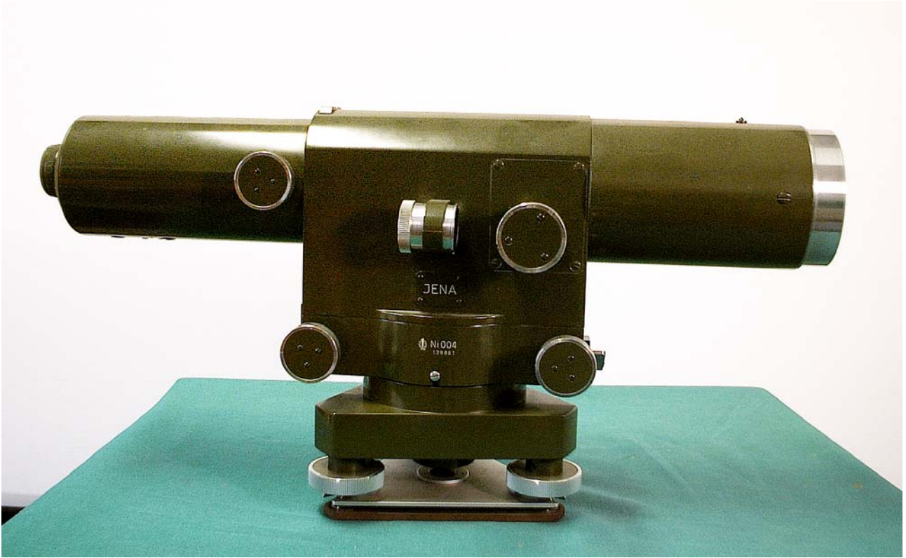
N° inventario 303 – Livello Zeiss Ni 004 matr.129861 (1960)
