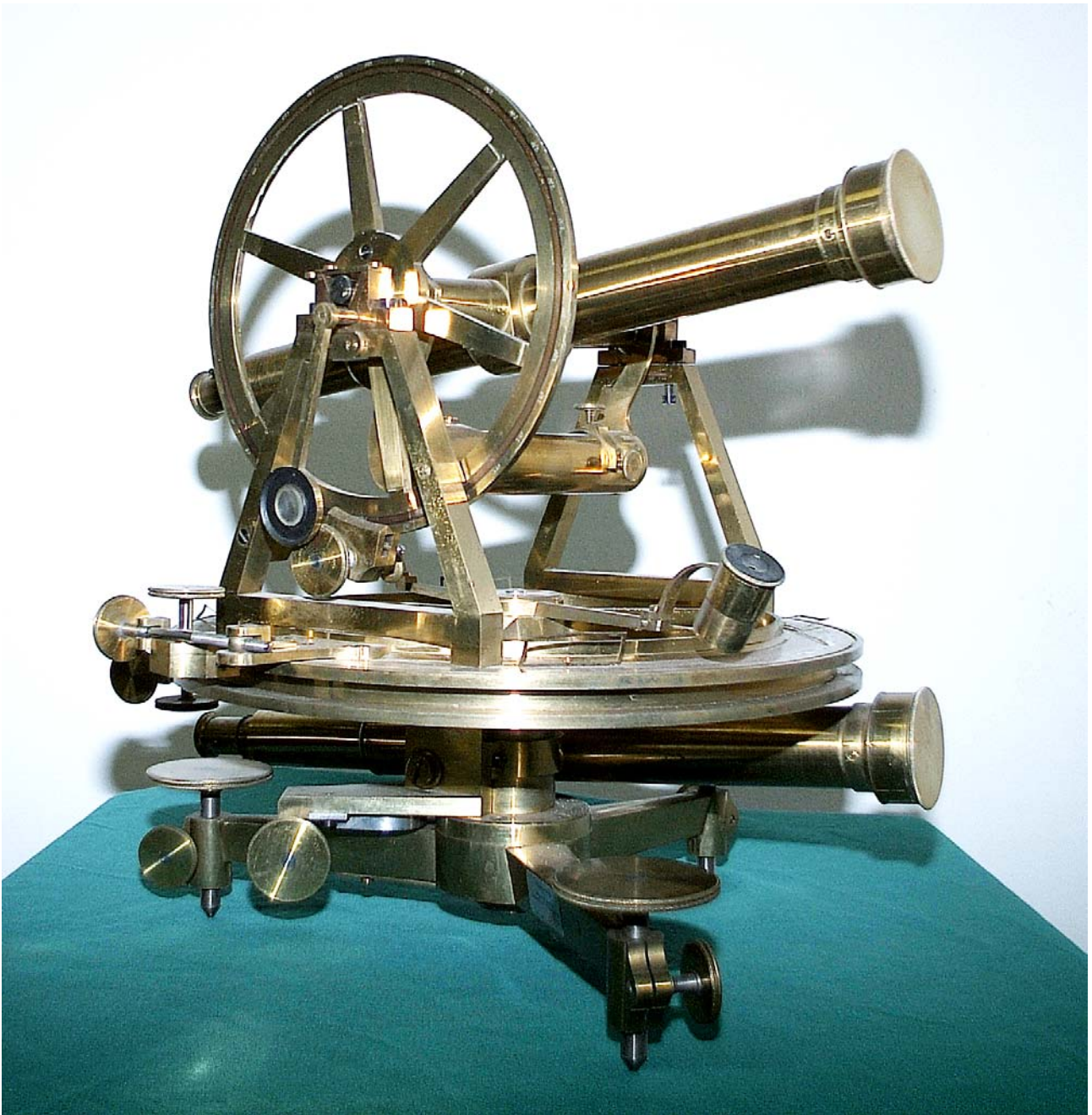
N° inventario 357 – Teodolite ripetitore di Reichenbach (1961)
