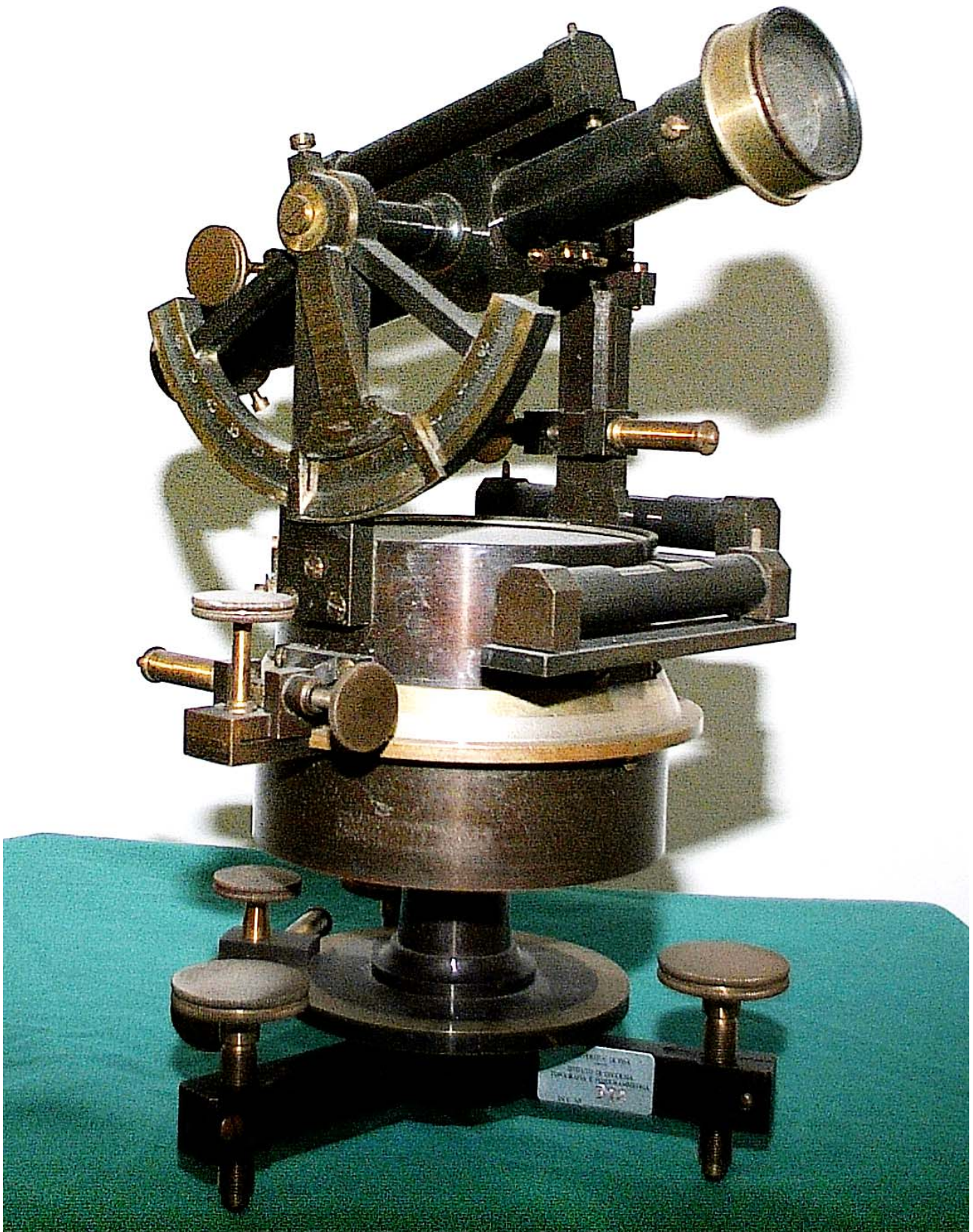
N° inventario 372 – Squadro graduato Bardelli con cannocchiale (1961)
