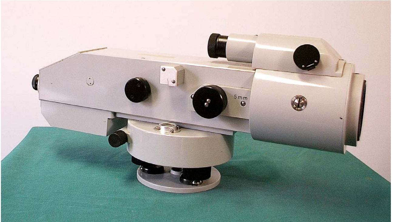
N° inventario CNR 375015 – Autolivello Zeiss Ni1 matr. 81491
