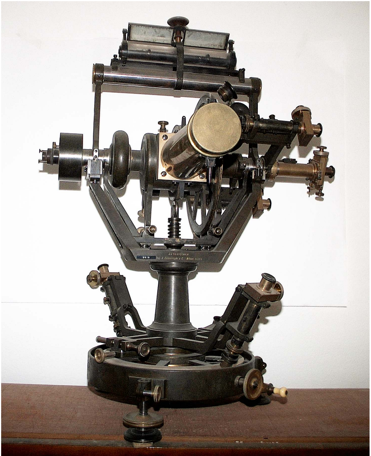
N° inventario 377 – Tacheometro Salmoiraghi per i passaggi (1961)
