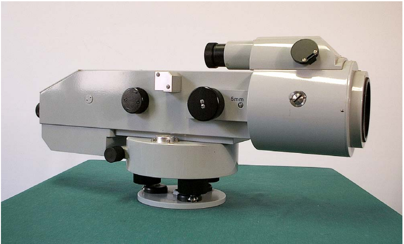
N° inventario CNR 385604 – Autolivello Zeiss Ni1 matr. 107384
