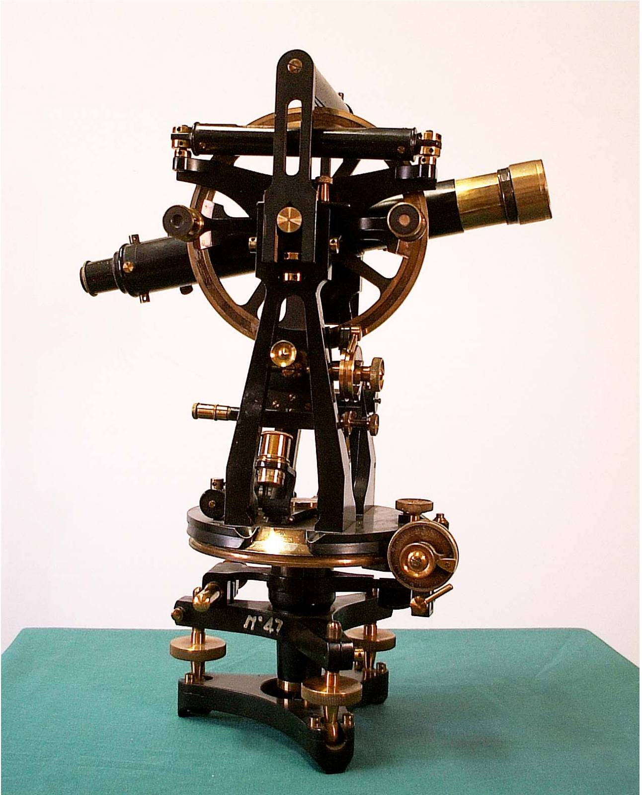
N° inventario 44 – Teodolite Casella con micrometro di Reeves (1920)
