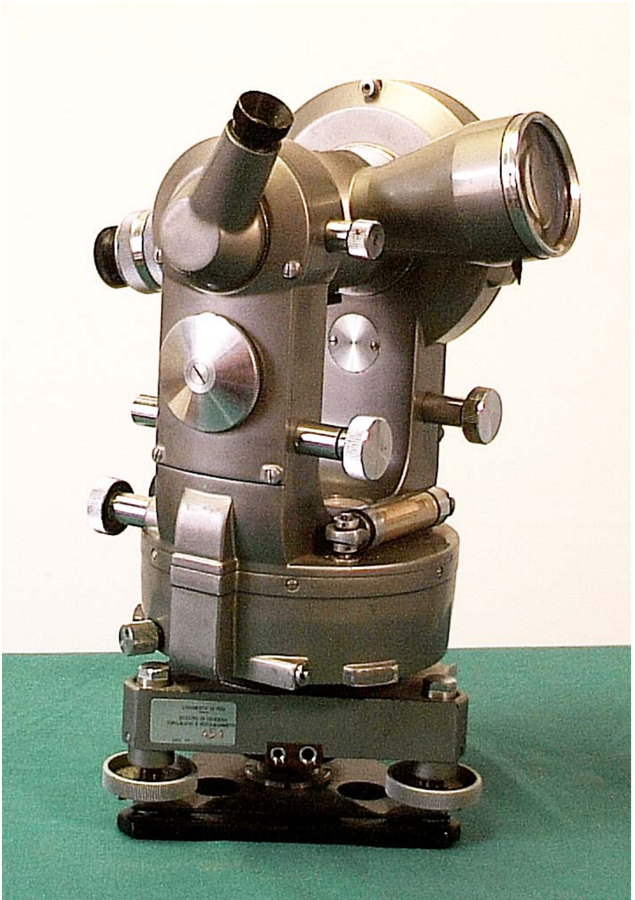
N° inventario 451 – Tacheometro Officine Galileo TG2b n. 01159 (1966)
