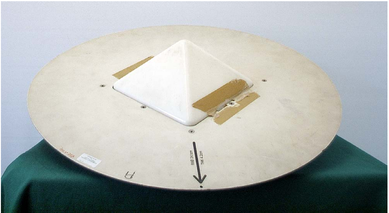
N° inventario 757 – Antenna per ricevitore GPS Trimble 4000 SL (1991)
