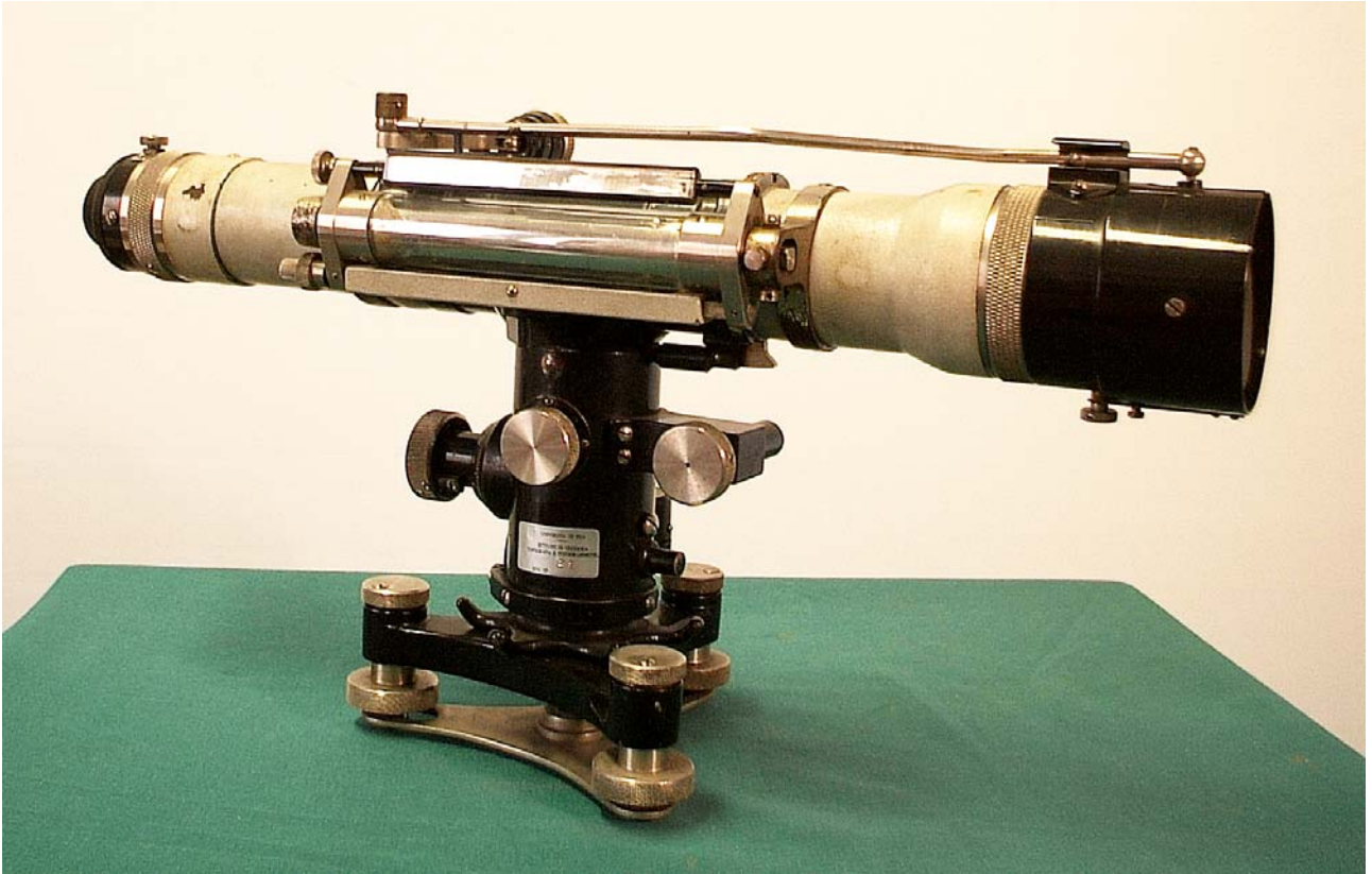
N° inventario 81 – Livello Zeiss mod. III matr. 4458 (1929)
