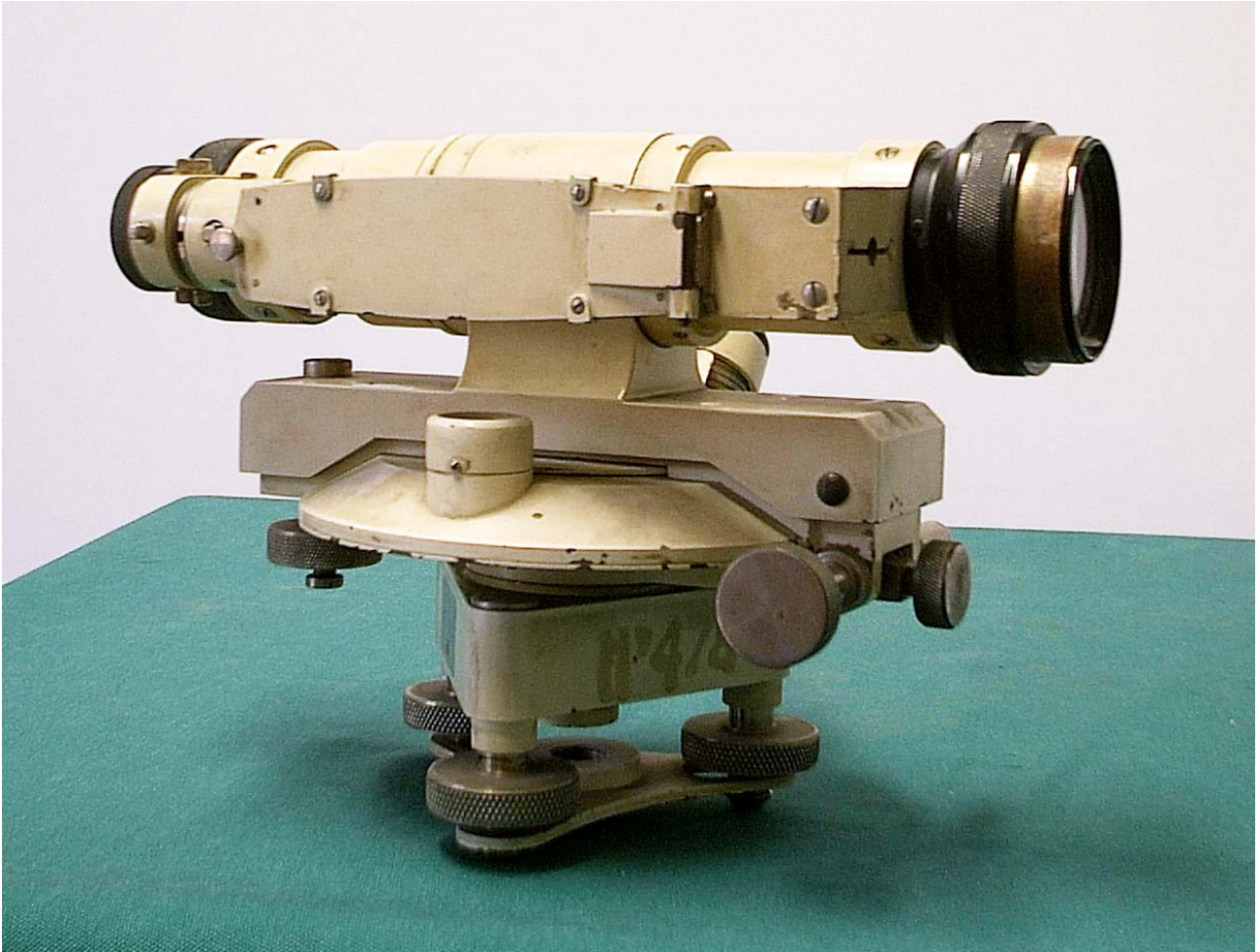
N° inventario 96 – Livello Salmoiraghi “a manicotto” mod. 5164 matr. 69941 (1936)
