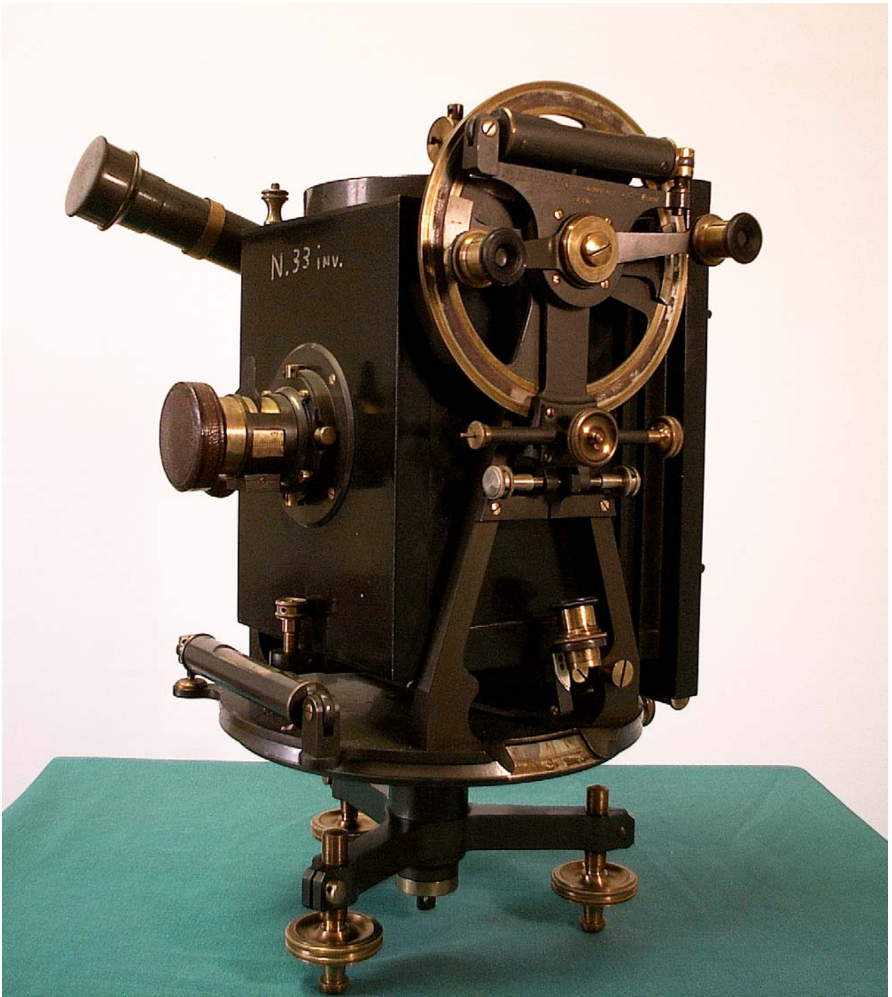
Tacheometro fotografico
